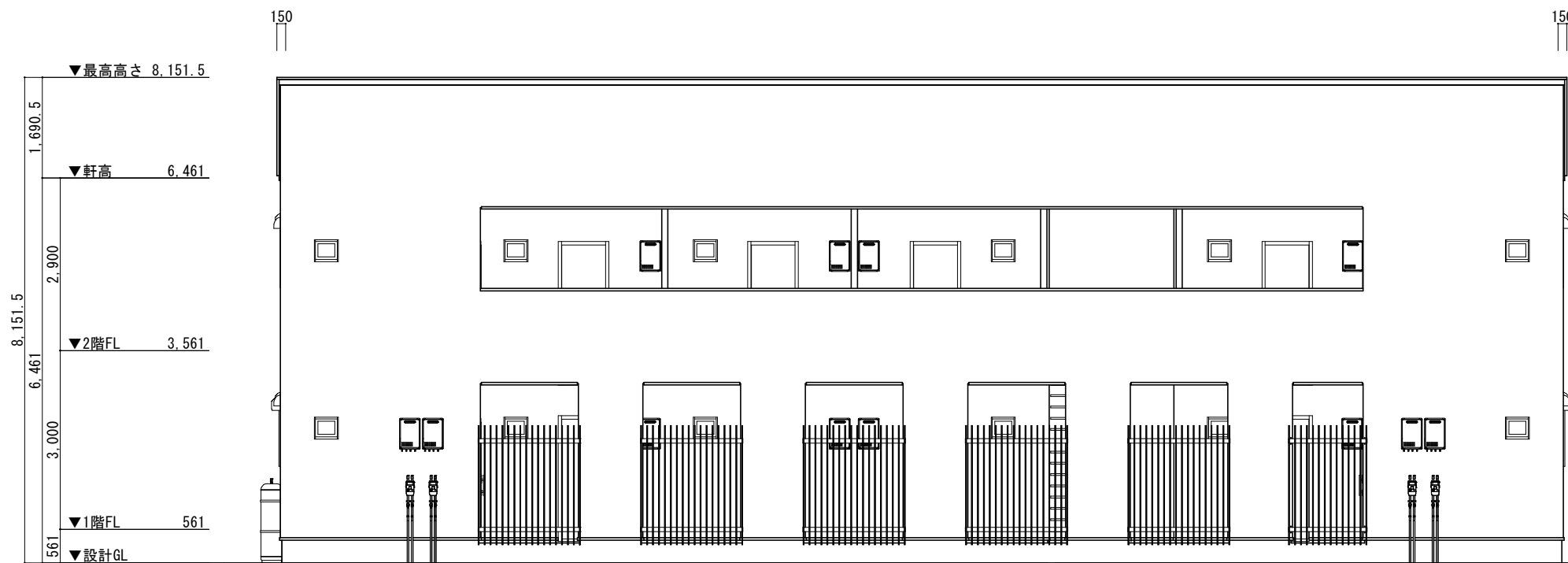
北立面図 S=1/100
