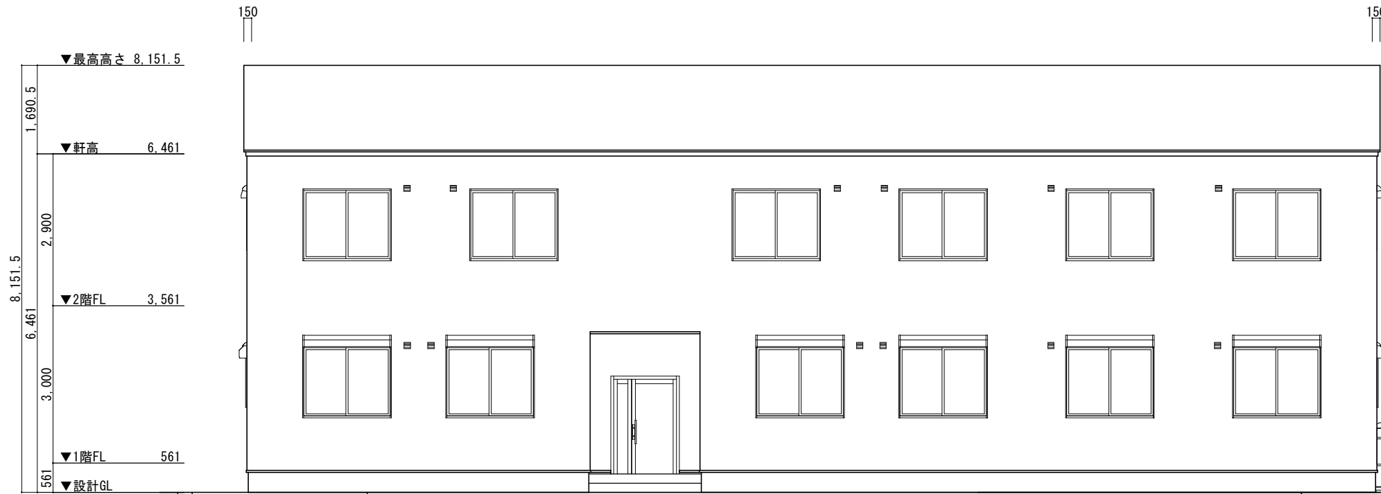
南立面図 S=1/100
