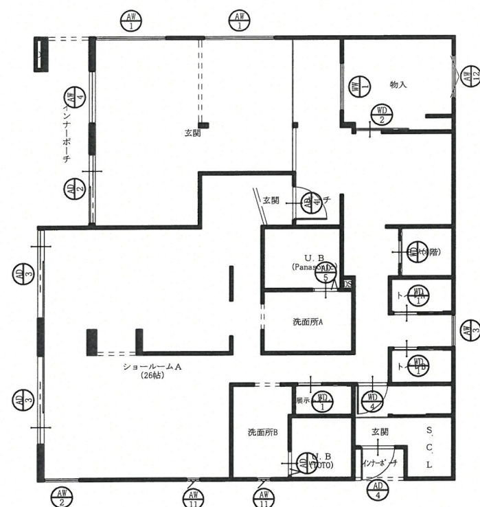
1階 建具配置図 S:1/150
