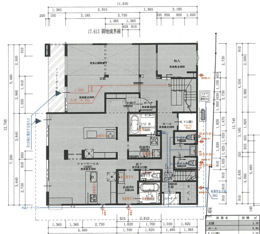
25.453 隣地境界線 1階 平面図 S:1/150
