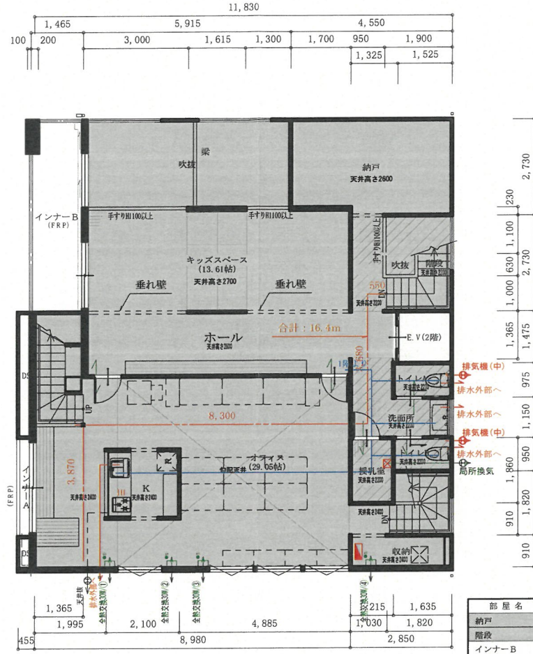
2階 平面図 S:1/150
