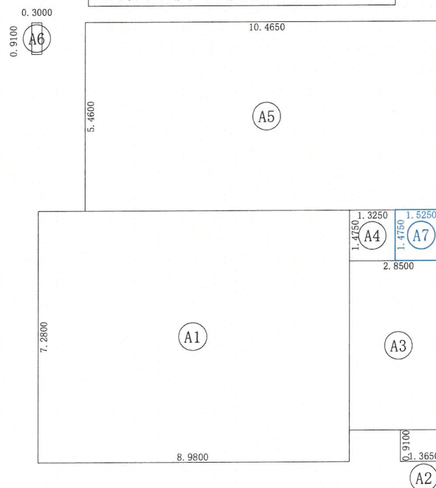
建築面積求積図 S:1/150
