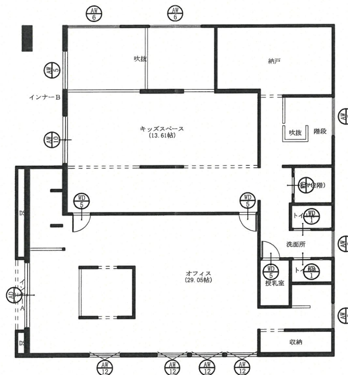
2階 建具配置図 S:1/150
