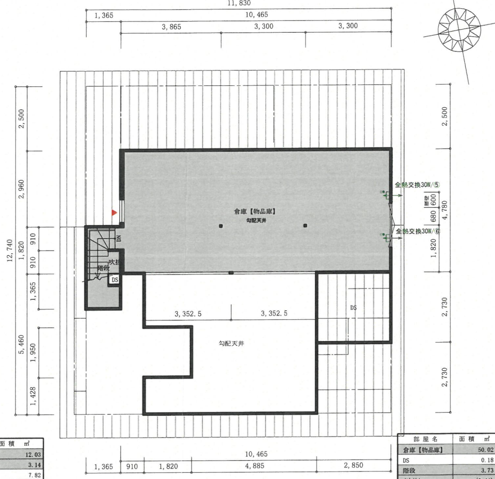
3階 平面図 S:1/150
