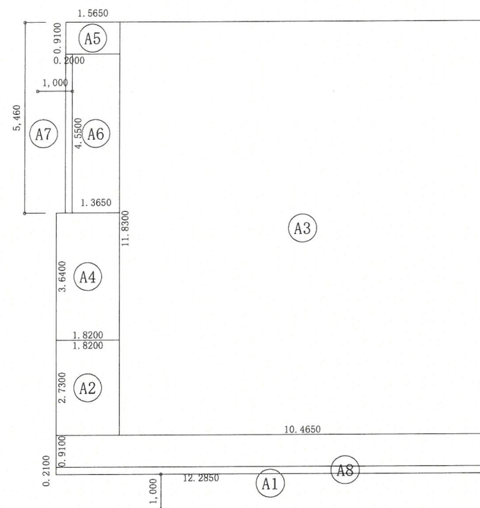
建築面積求積図 S:1/150
