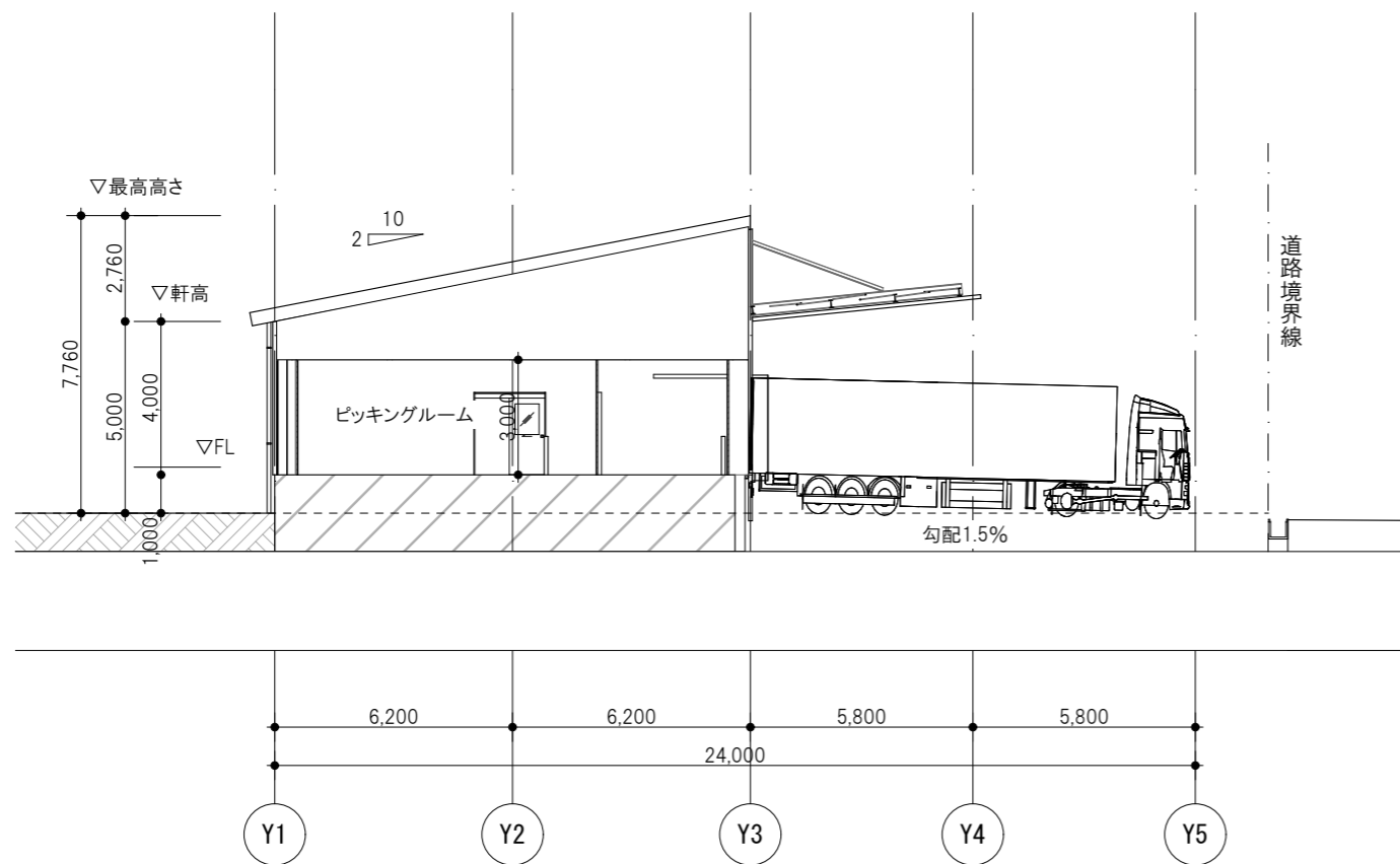
断面図 1:200
