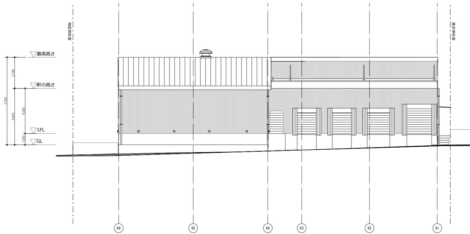
北立面図 1:200
