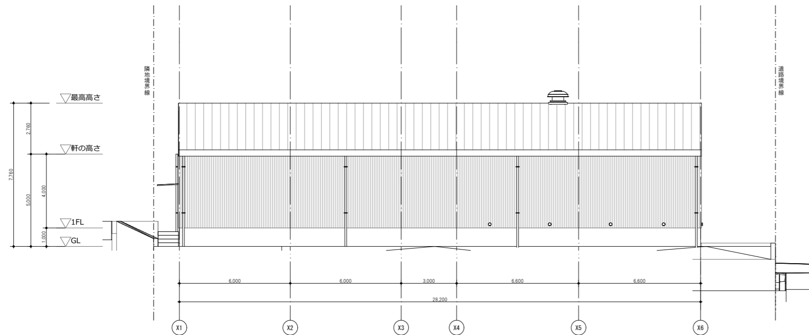
南立面図 1:200
