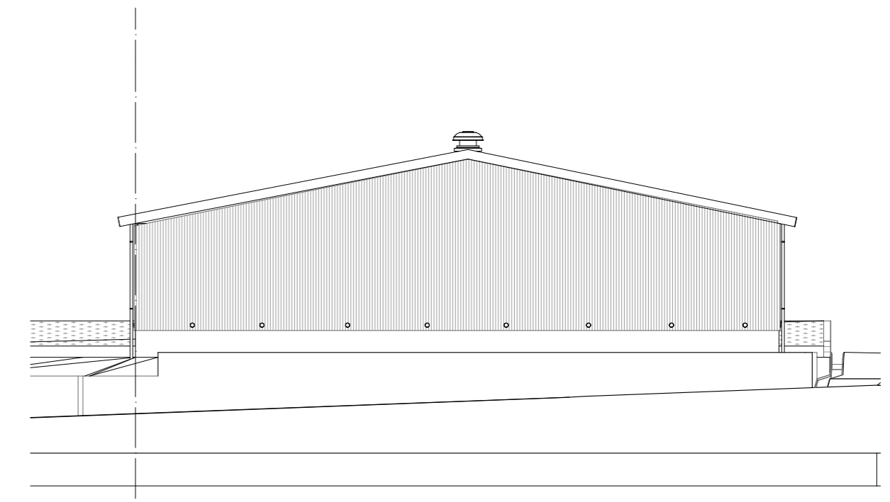
東立面図 1:200
