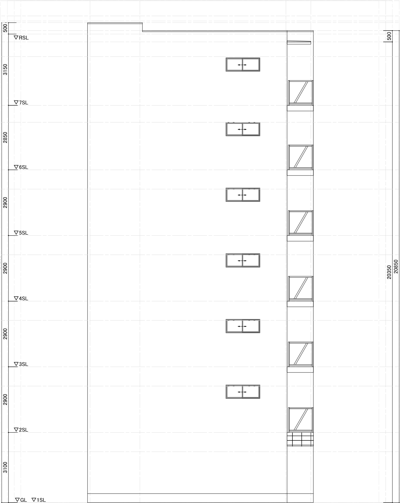
東立面図
