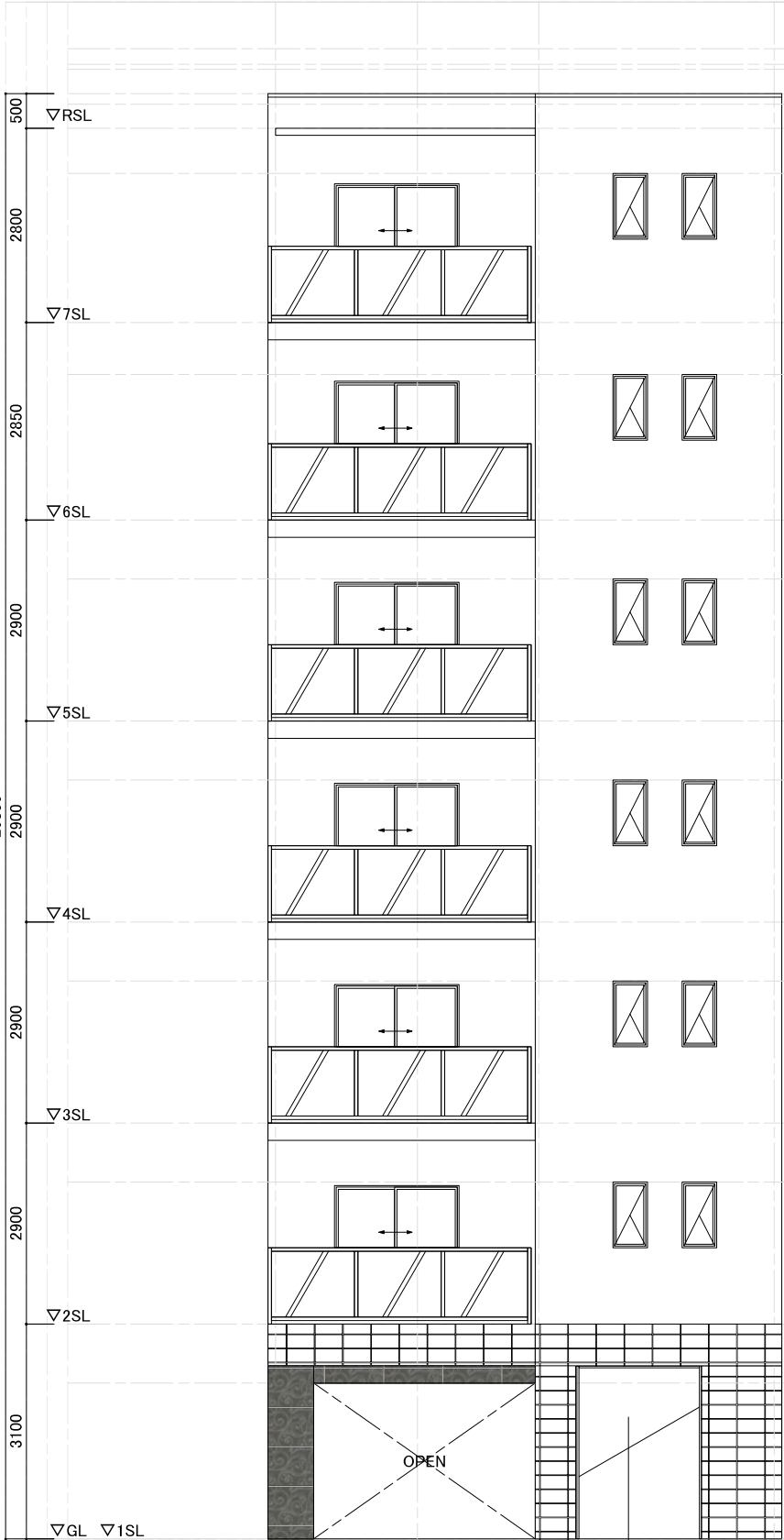
北立面図
