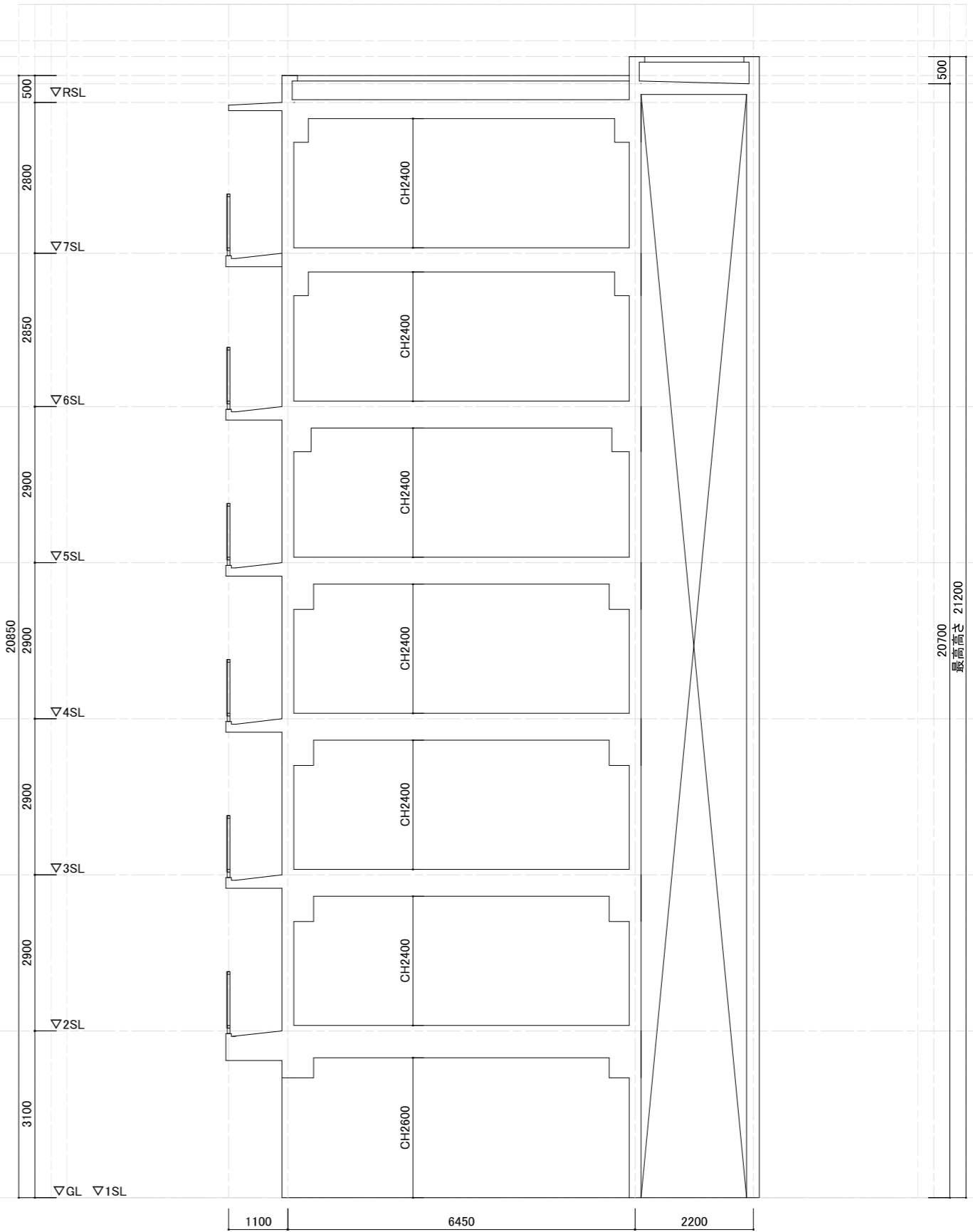
西立面図
