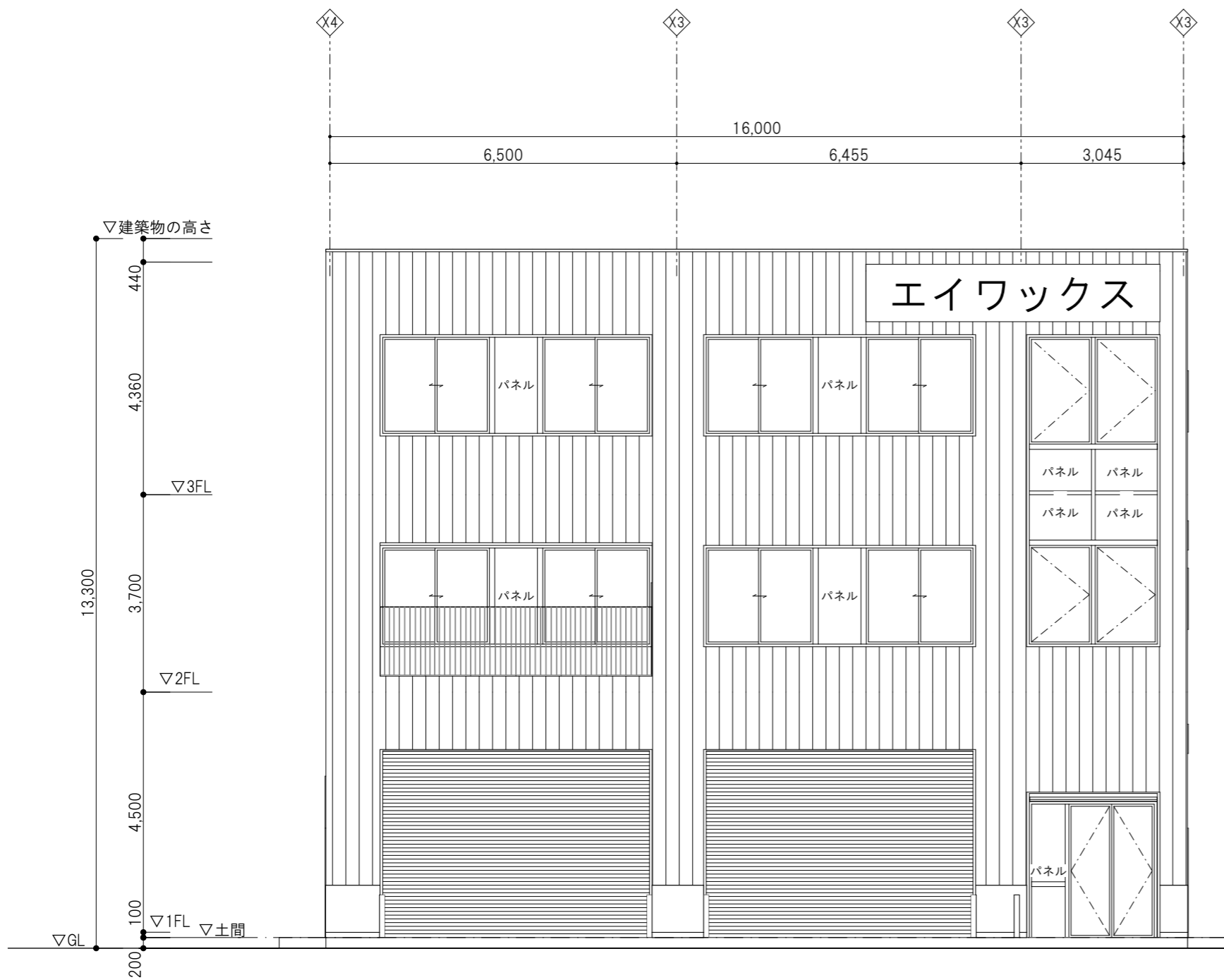
北立面図 1:100
