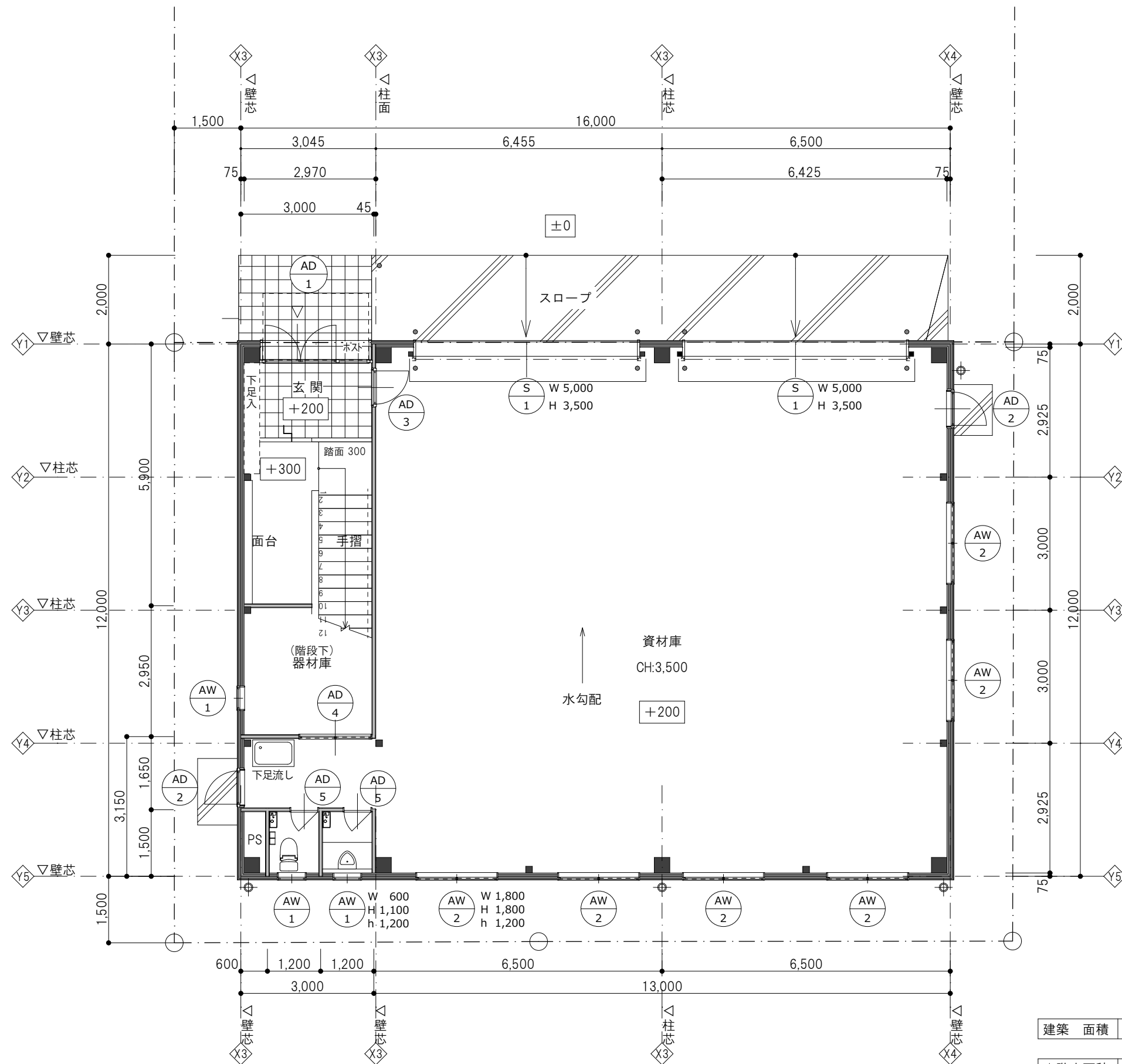
1階平面図 1/100
