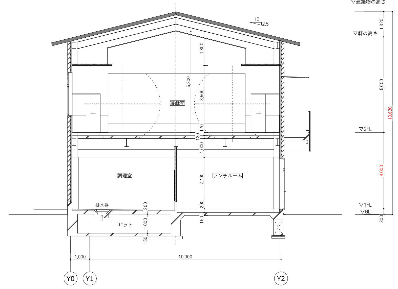
X2 断面図
