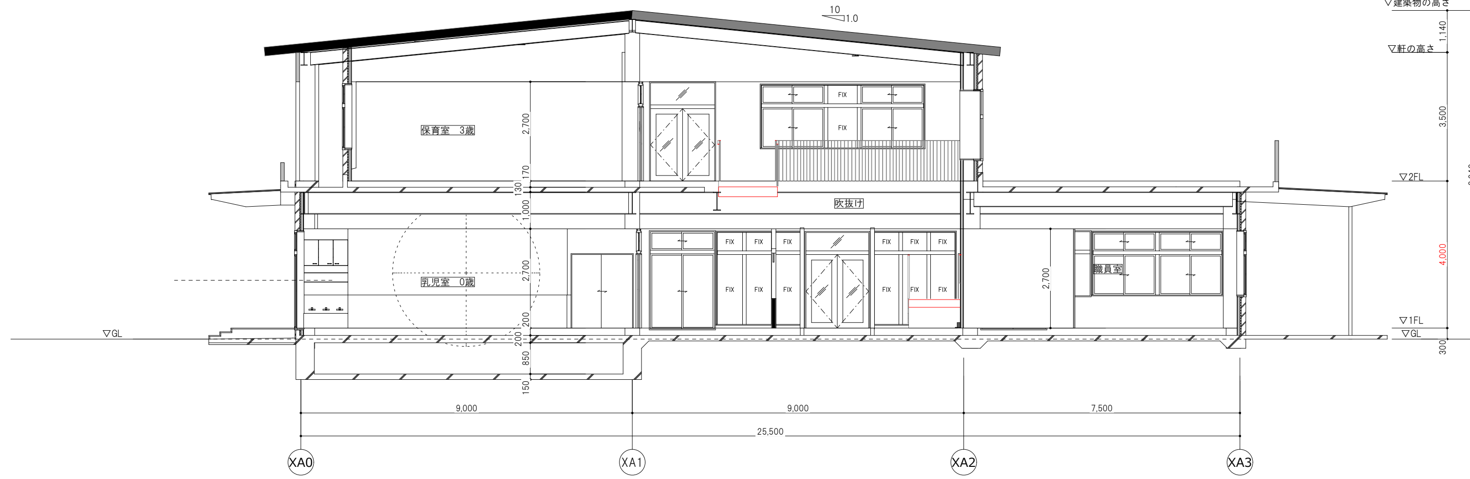
Y1 断面図
