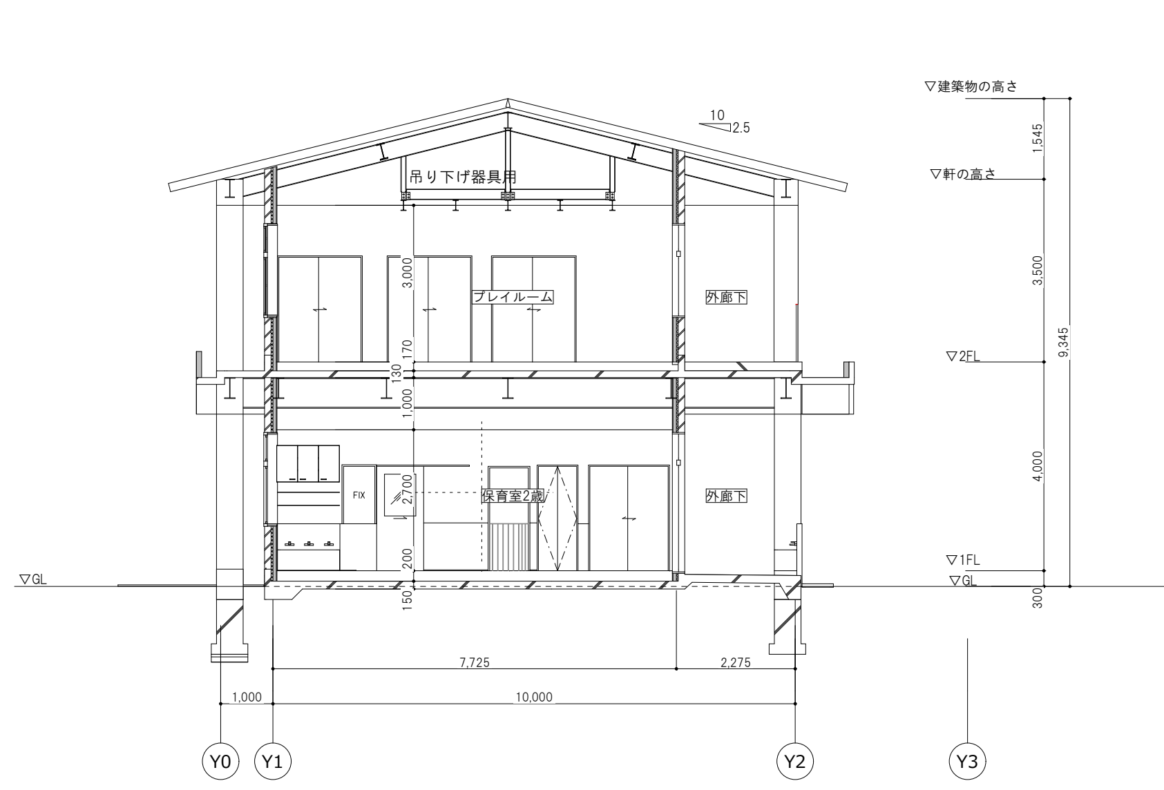
X1 断面図
