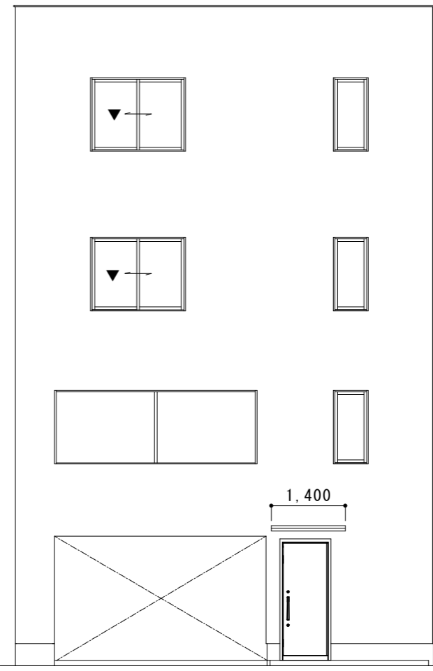
南側立面図
