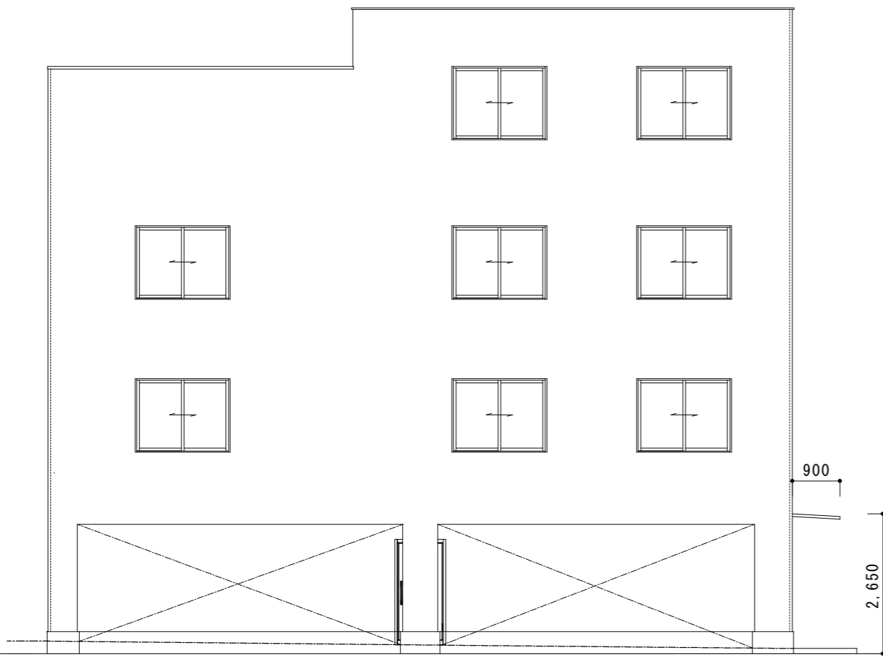
西側立面図
