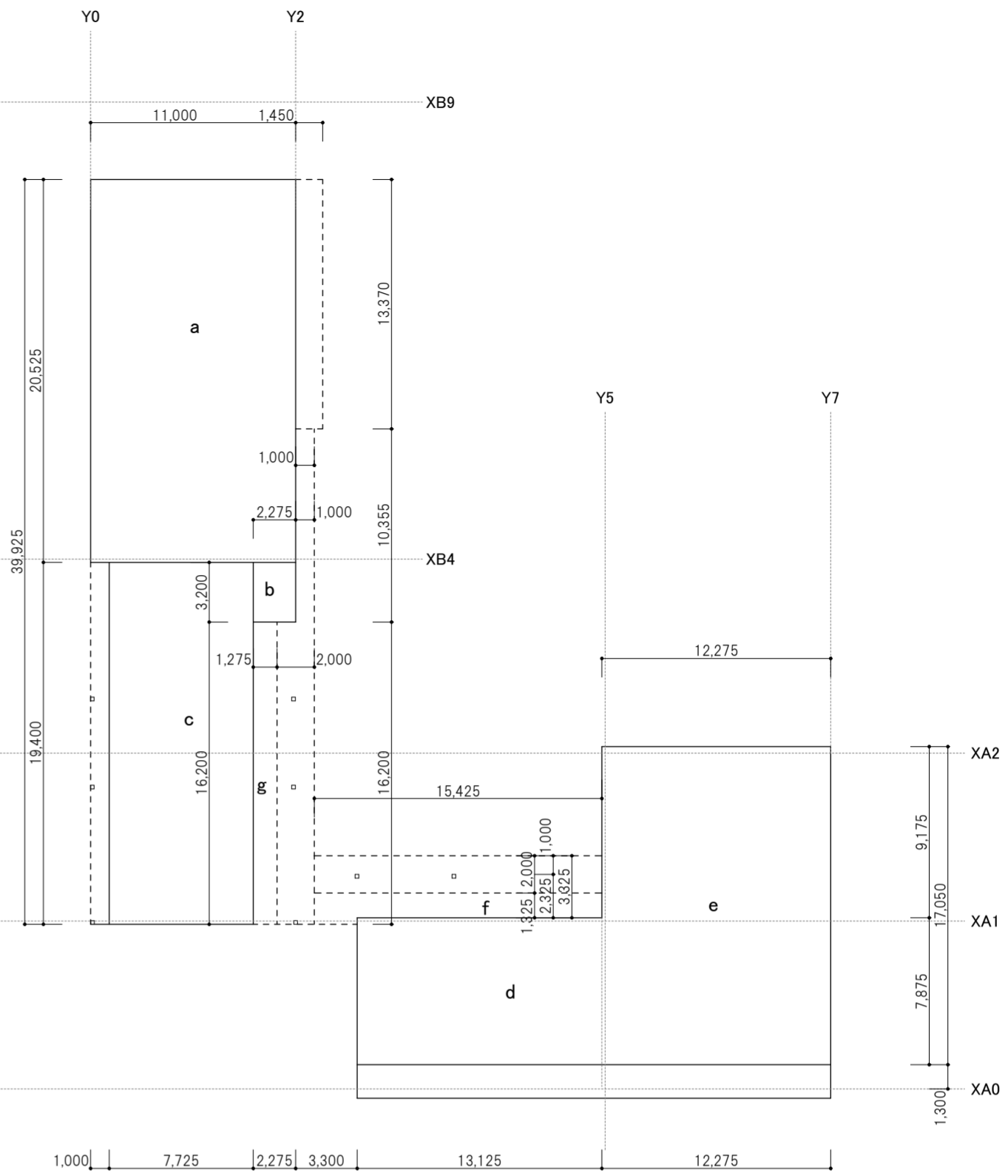
2階床面積求積図 1/300
