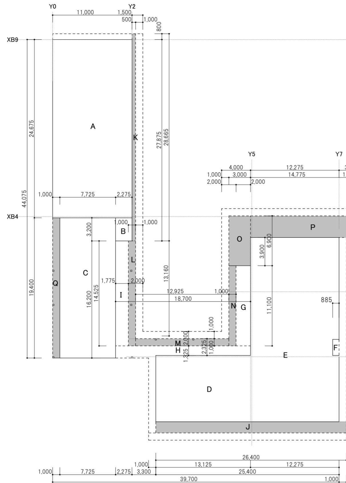
1階床面積求積図 1/300
