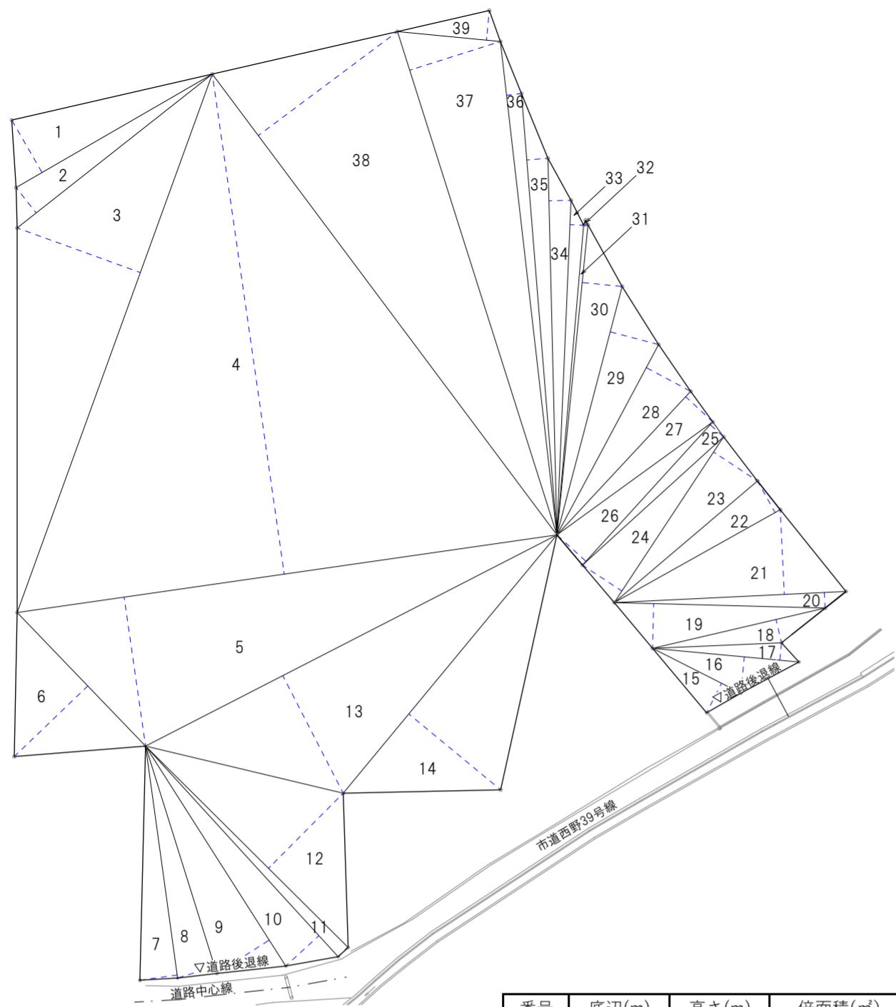
敷地面積求積図 1/500
