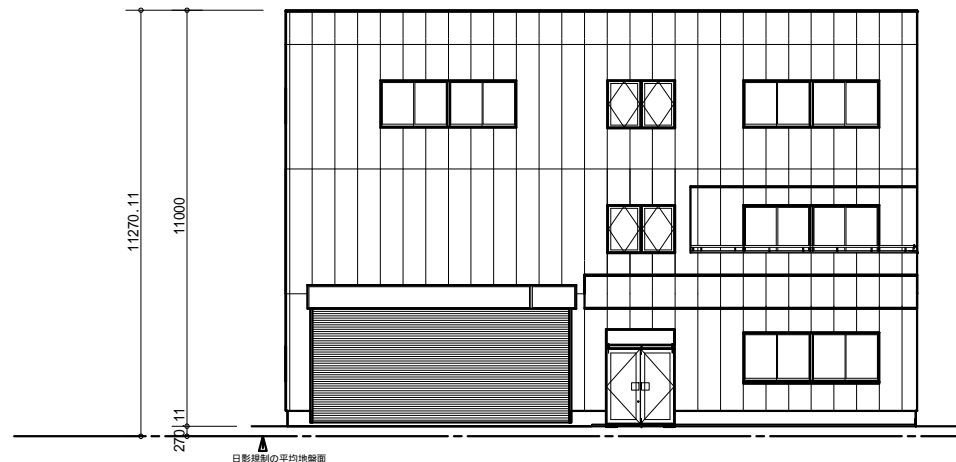
北側立面図 1/200
