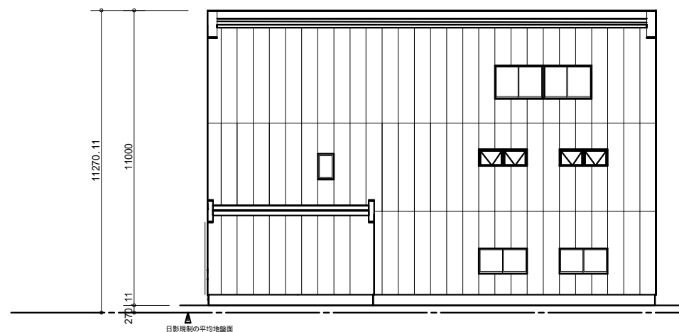
南側立面図 1/200
