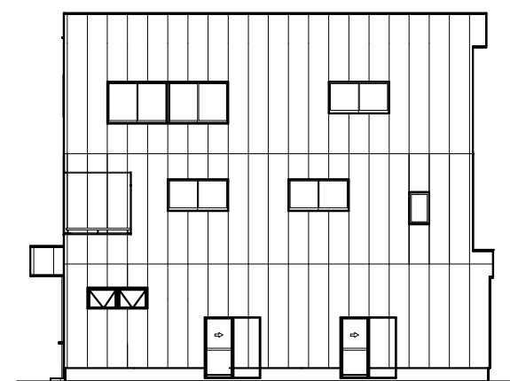
西側立面図 1/200
