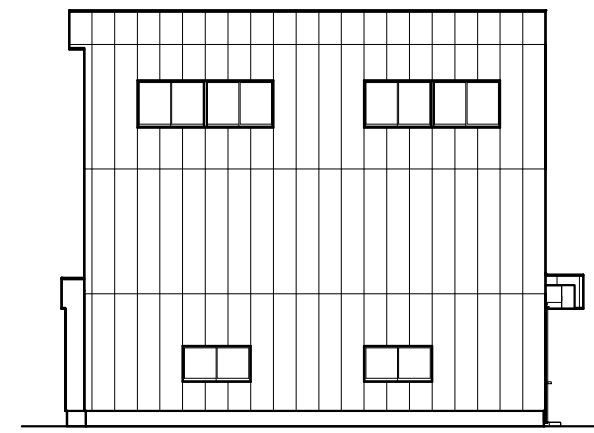
東側立面図 1/200
