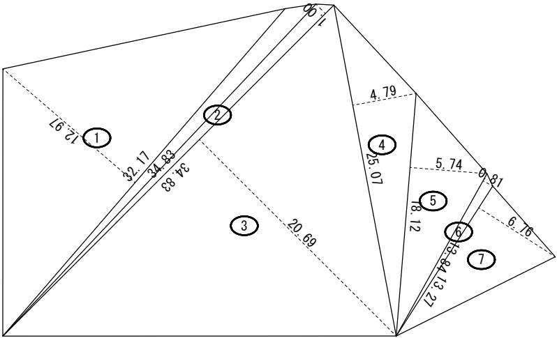
敷地求積図 S-1/400
