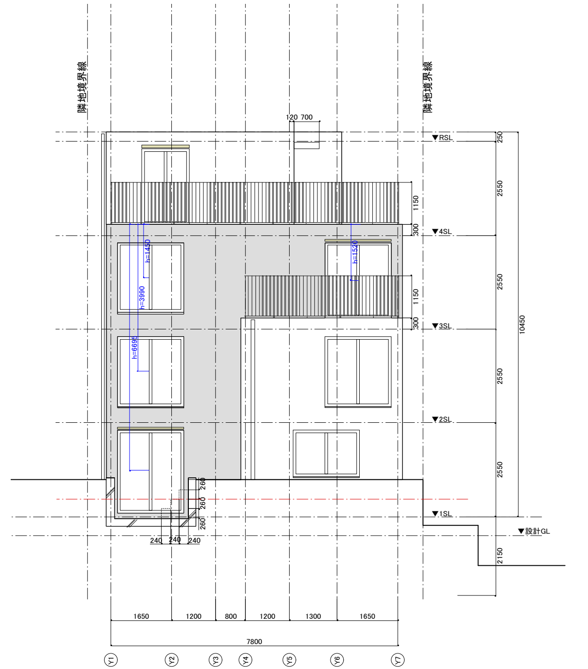
東側立面図
