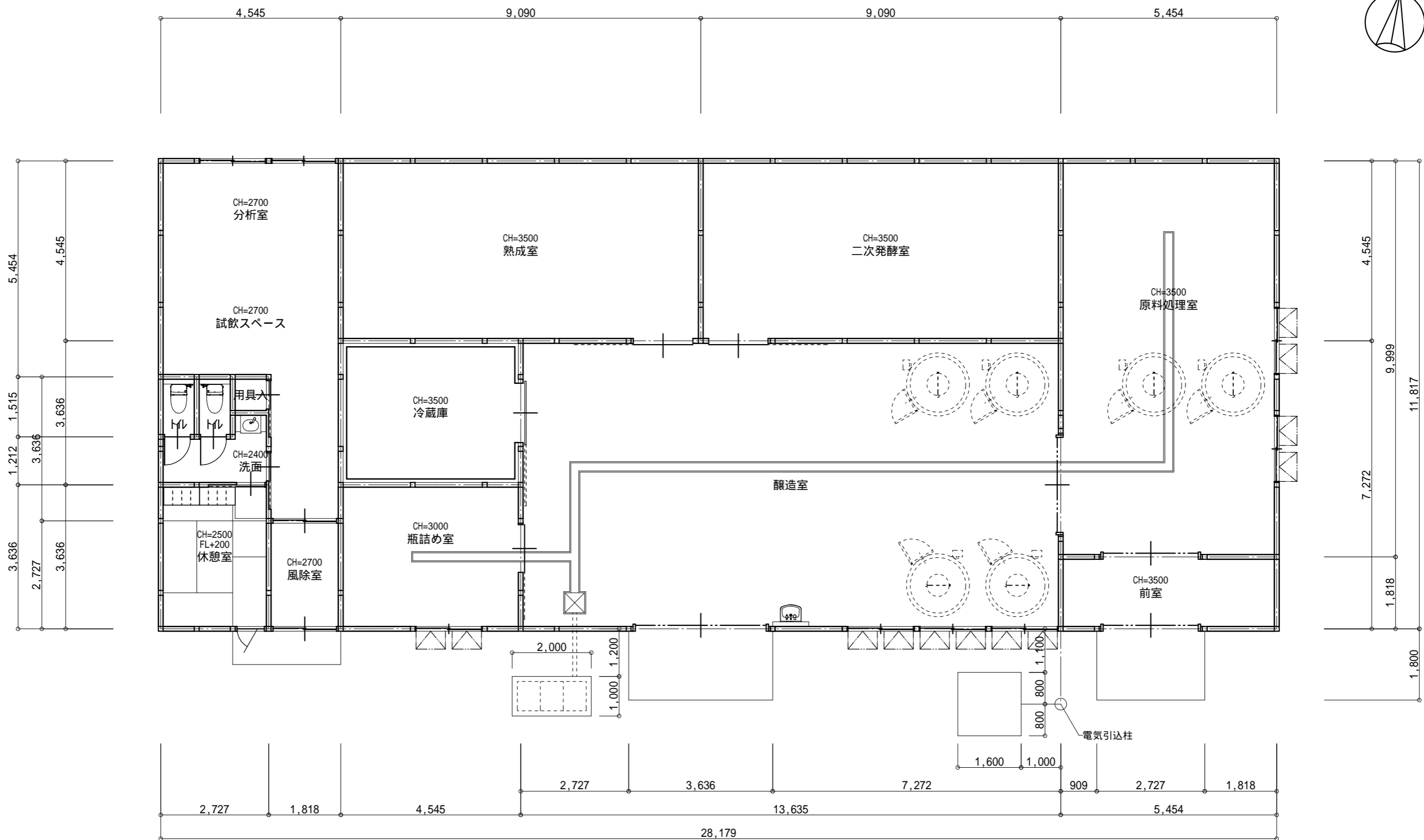
平面図 S-1/100 延べ床面積 = 332.99㎡
