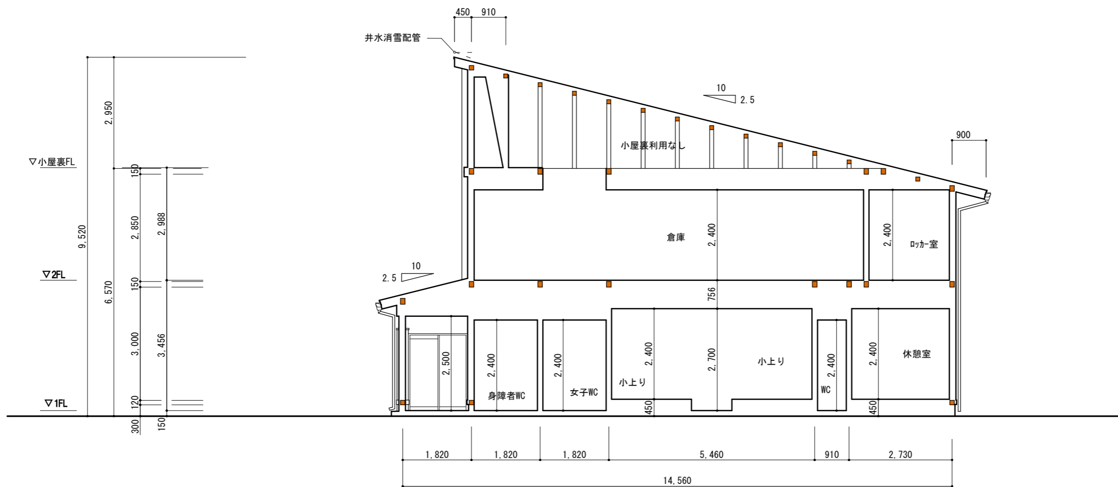
断面図 1 S=/100
