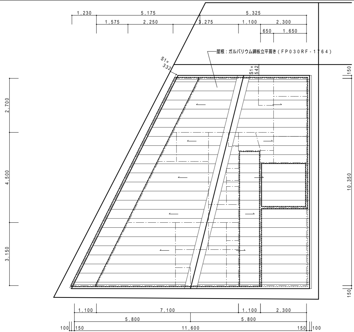
屋根伏図 S=1:100
